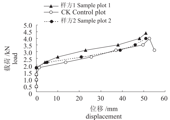
图1 不同样方载荷与位移的关系
